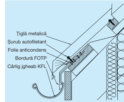
LTM 300 Înclinație acoperiș între 24° și 90°
