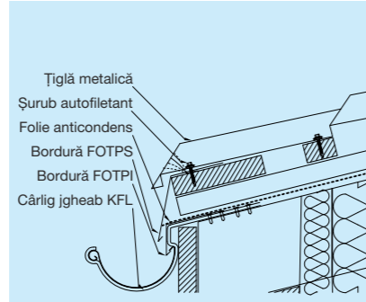
LTM 300 Înclinație acoperiș între 14° și 90°
