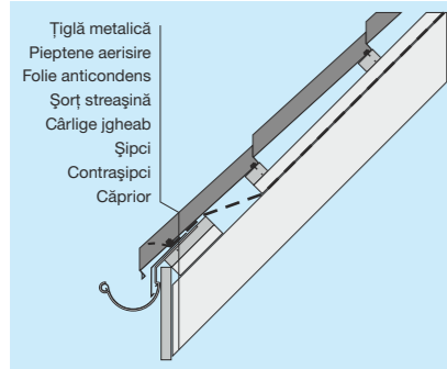
Nordic 400 / Skane Înclinație acoperiș între 14° și 90°
