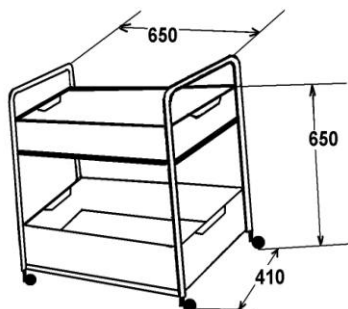
CARUCIOR 2.15 CU 2 COSURI 650X410X650
