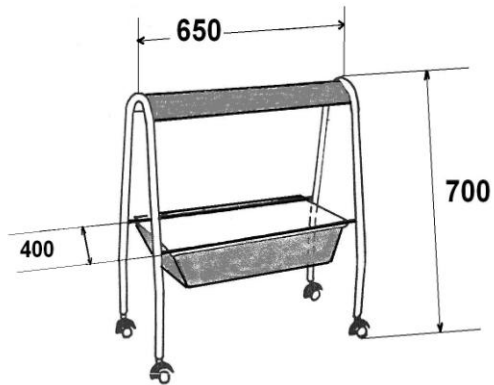
CARUCIOR 2.4 700 X 650 X 400
