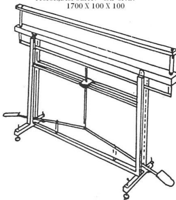
DISPOZITIV DE FIXARE A FOILOR DE SPAN LA CAPETE, CU ACTIONARE LA PICIOR, DISPOZITIV "CAP SPAN" 1700 X 100 X 100
