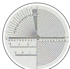
Nr. 6: Scala universală Art. Nr. 0135-101
