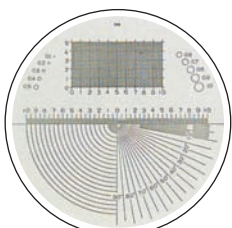
Nr. 4: Scala universală Art. Nr. 0135-089
