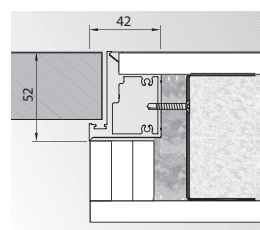
falț ascuns (deschidere spre interior)
