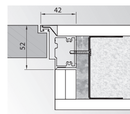
fără falț (deschidere spre exterior)
