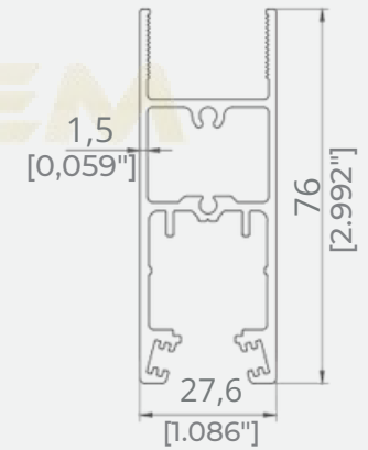
PROFIL BAZĂ PANOUL STICLĂ 22 MM
